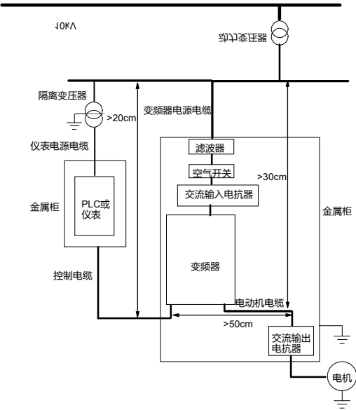
图 4-5 变频器的安装示意图
