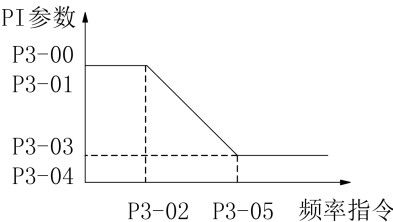
图 6-7 PI 参数示意图
