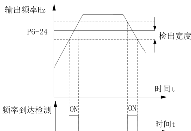
图 6-13-2 频率到达检出幅值示意图
