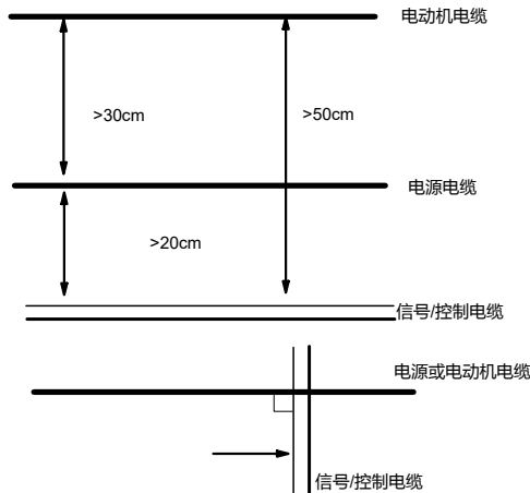
图 4-14 系统配线要求
