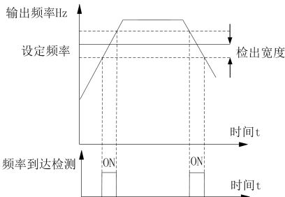
图 6-13-1 频率到达检出幅值示意图
