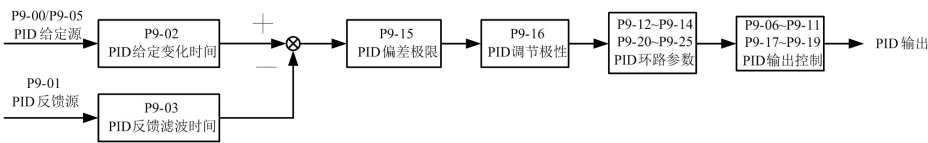
图 6-15 过程 PID 原理框图
