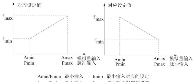
图 6-12 模拟/脉冲给定与设定量的对应关系
