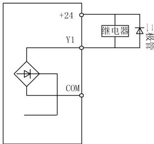
图 4-13 数字输出端子接线示意图
