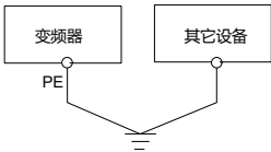
图 4-18 接地示意图 2
