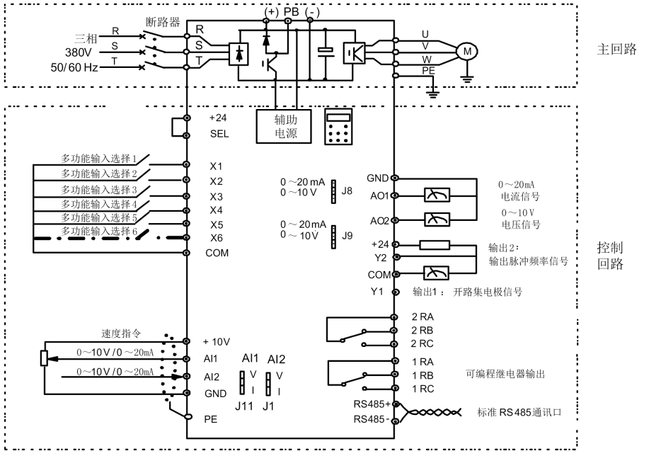
图 4-7 基本配线图
