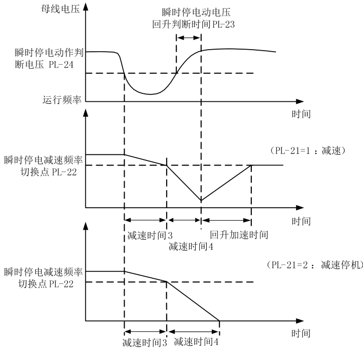
图 6-29 瞬时停电动示意图
