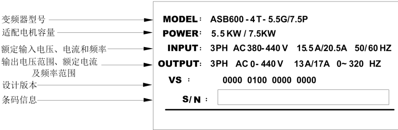
图 3-2 变频器铭牌
