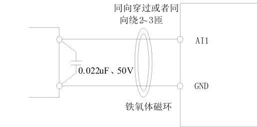
图 4-9 模拟量输入端子处理接线图
