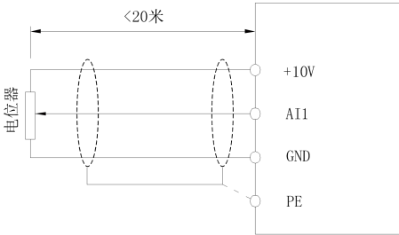
图 4-8 模拟量输入端子接线示意图
