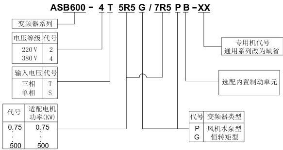
图 3-1 变频器型号
