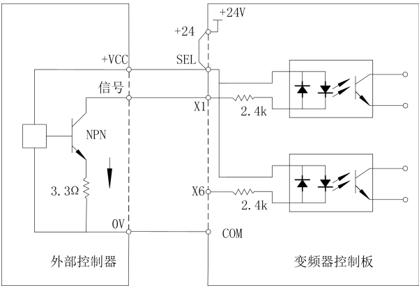
图 4-10 漏型接线方式
