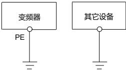
图 4-17 接地示意图 1
