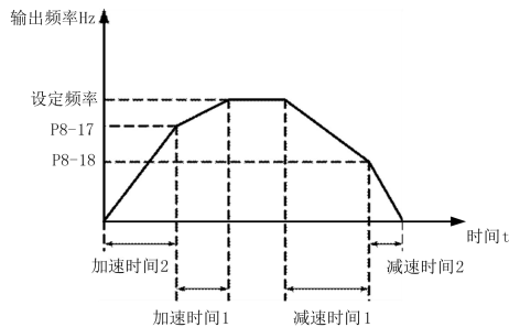
图 6-21 加减速时间切换示意图
