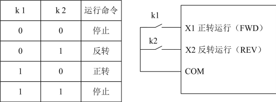
图 6-8 两线式模式 1
