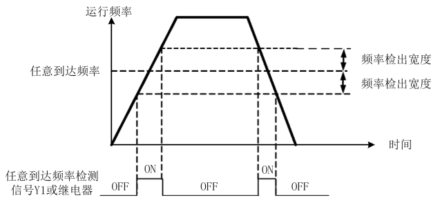
图 6-24 任意到达频率检测示意图
