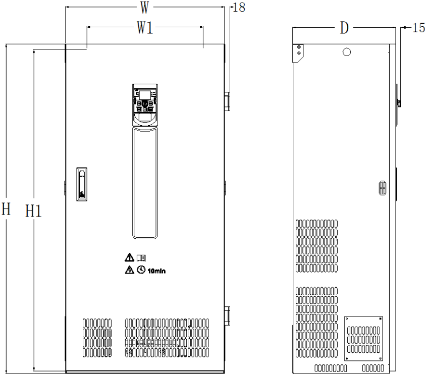
图 2-6. 160KW 以上变频器外型尺寸及安装尺寸示意图
