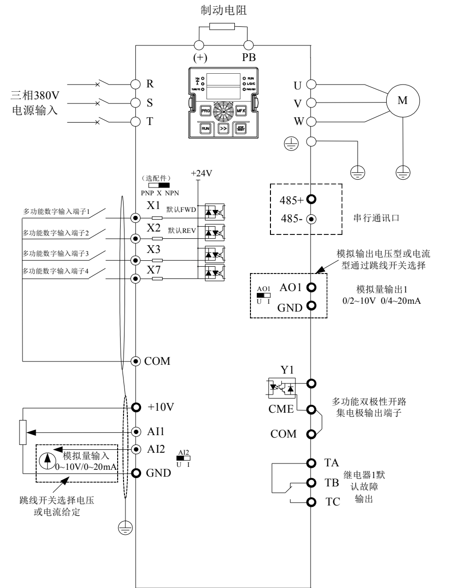
图3-1. 三相380V 2.2kW (4T:380V) 及单相220V (2S) 1.5kW(输入接L N或R T)以下变频器接线图 备注：数字输入端子X跳线开关出厂默认NPN模式（即X短接COM有效），PNP模式为选配功能，三相380V 2.2 kW 及单相220V 1.5 kW 以下如需选配PNP模式，订货时请说明。AI2, AO1跳线开关出厂默认电压模式。
