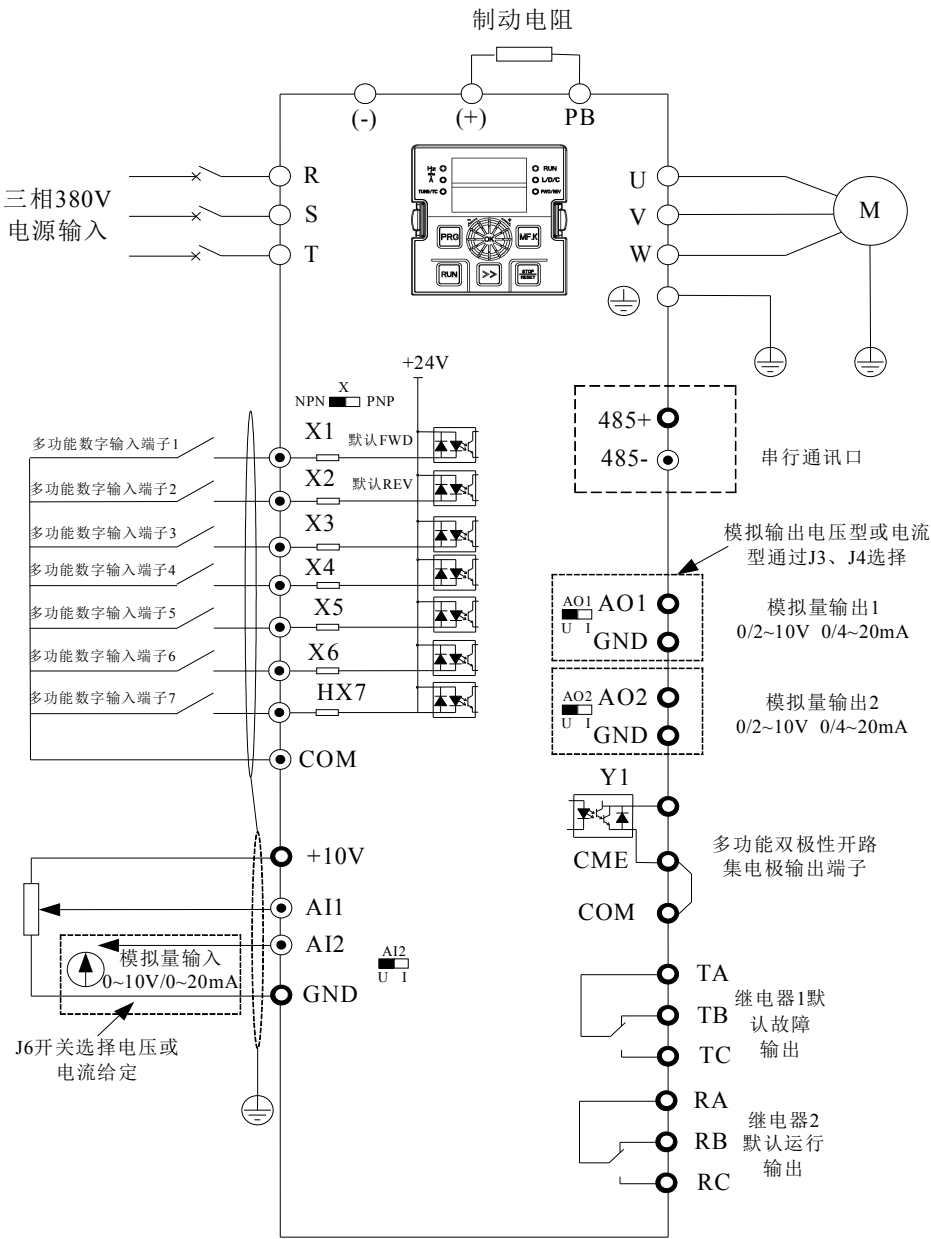
图 3-2. 三相 380V 4.0~ 30kW (4T:380V) 及单相 220V (2S) 5.5kW 以下(输入接 R T)变频器接线图 备注: 数字输入端子 X 跳线开关出厂默认 NPN 模式(即 X 短接 COM 有效), AI2, AO1, AO2 跳线开关出厂默认电压模式。
