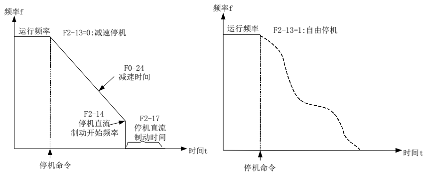
图4-13. 停机示意图
