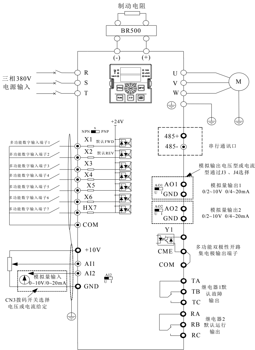
图 3-3. 三相 380V 37 ~ 75 kW (4T:380V) 变频器不带制动单元功能接线图 备注：数字输入端子 X 跳线开关出厂默认 NPN 模式（即 X 短接 COM 有效），AI2, AO1, AO2 跳线开关出厂默认电压模式。ASB630/ASB630S 系列 37~110kW 制动单元部分属选配功能，如有需求，订货时请说明，选配了制动单元功能的接线图参考图 3-2。
