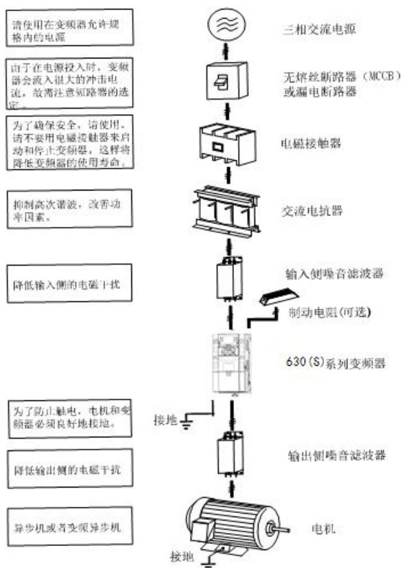
图 1 与外围机器的连接示例
