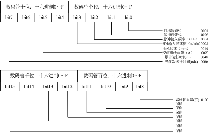
图 5-18. LED 运行显示位对应图
