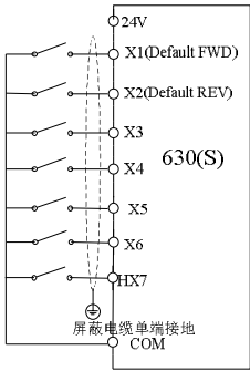
X接线模式一（出厂默认接线方式）：当X拨码开关为PNP模式没有使用外部电源
