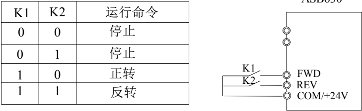
图5-8. 两线式运转模式2
