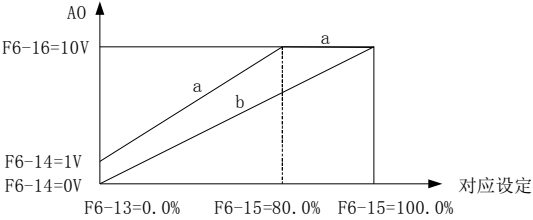
图4-29. F0输出示意图
