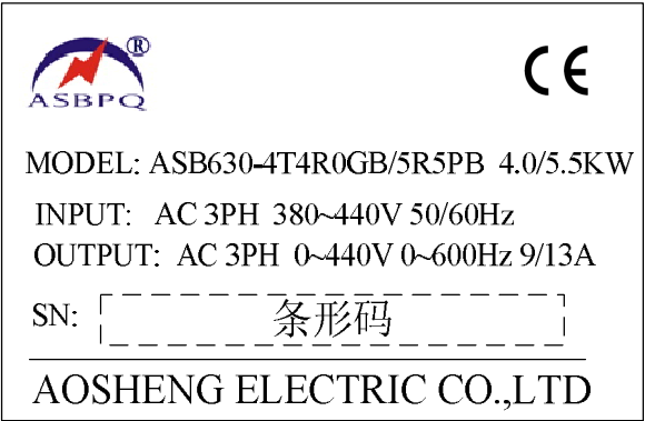
图2-2. 铭牌
