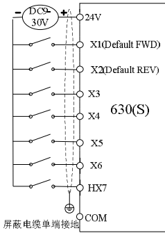
X接线模式二：当X拨码开关为NPN模式使用外部电源
