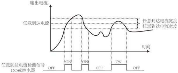
任意到达频率检测示意图
