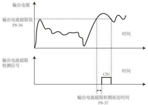
输出电流超限检测示意图
