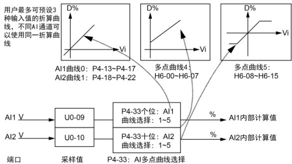
图6-20 AI信号对应实际给定
