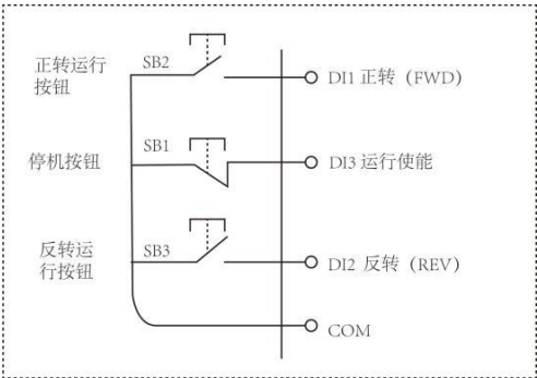
三线式控制模式1
