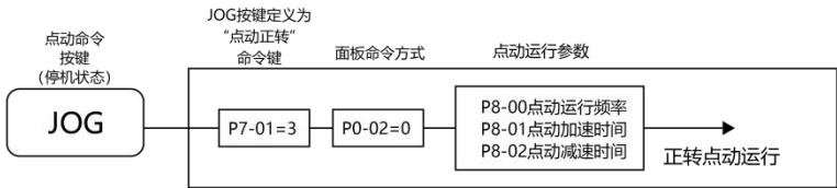
操作面板点动运行
