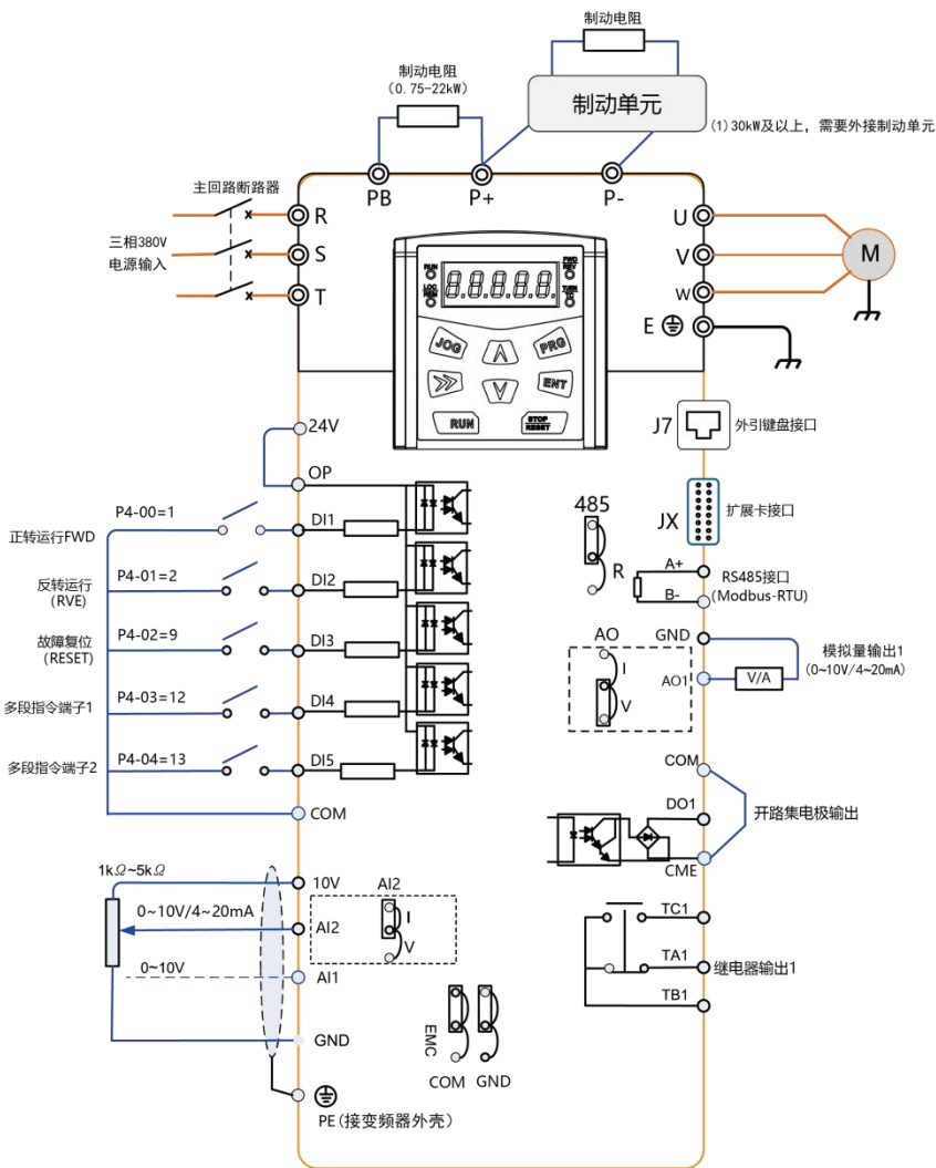
驱动器接线
