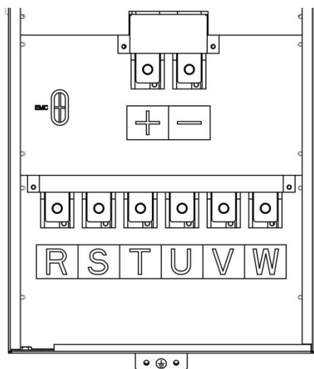
A10主回路接线端子
