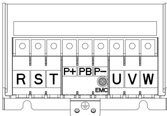
A3~A5主回路接线端子
