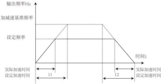
加减速时间示意图
