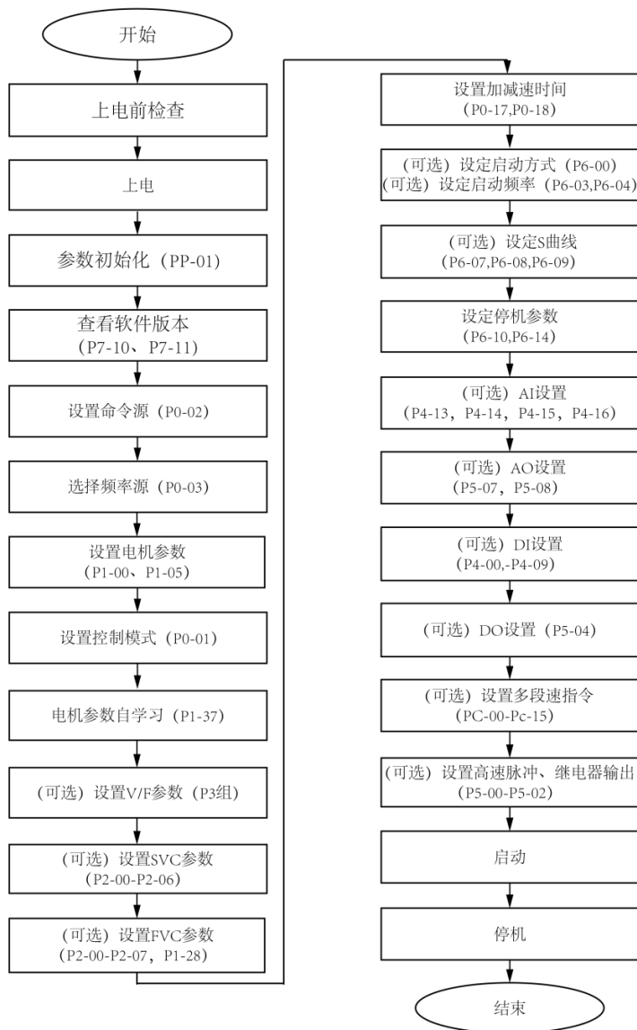
图7-1 基本调试流程
