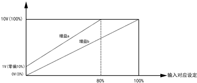
图6-21 AO输出示意图
