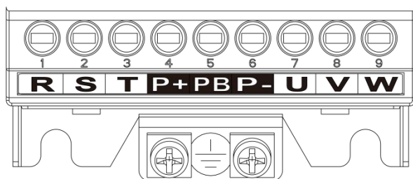
A1~A2主回路接线端子
