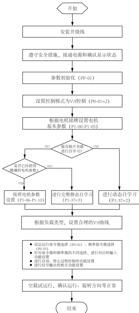
图7-2 V/F调试流程
