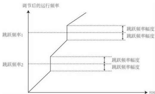
加减速过程中跳跃频率有效示意图
