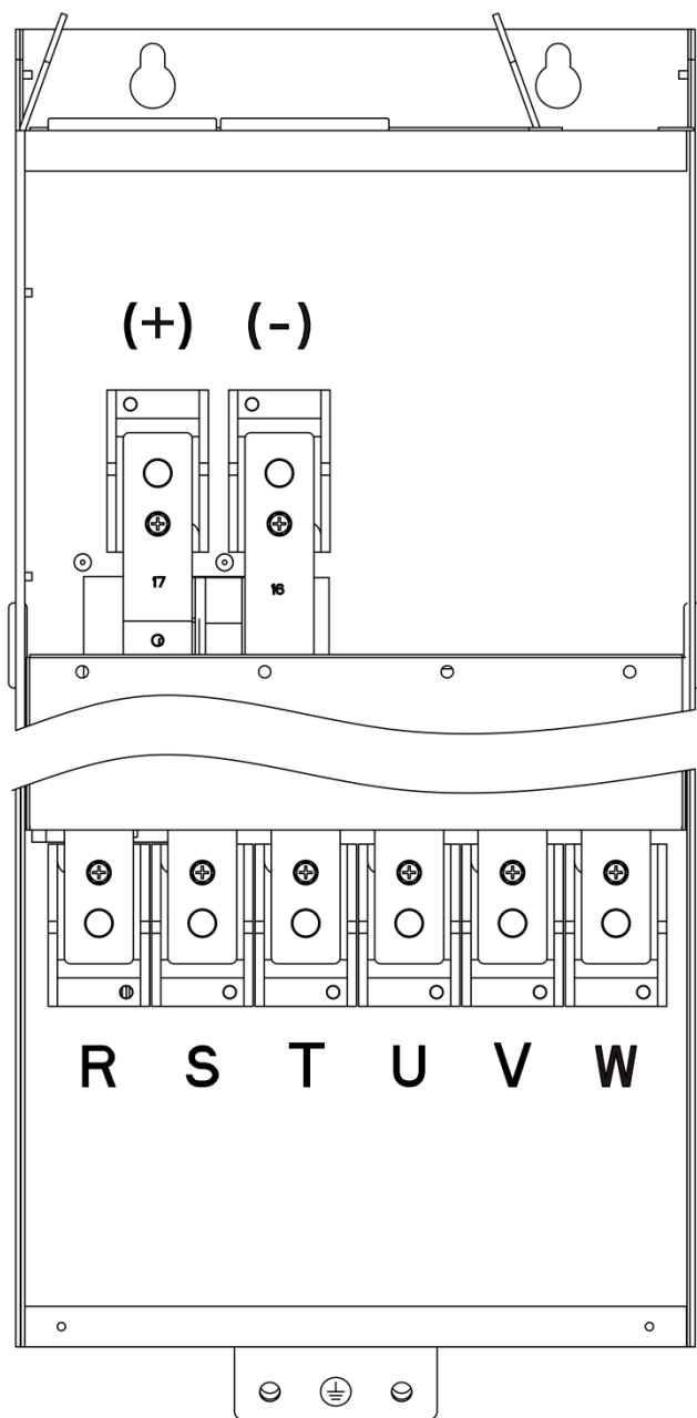
A11主回路接线端子
