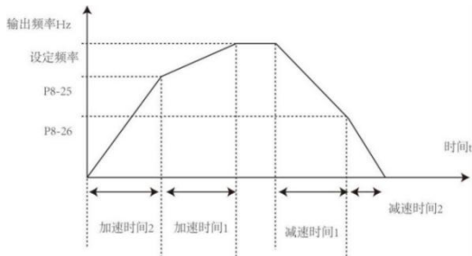
加减速时间切换示意图
