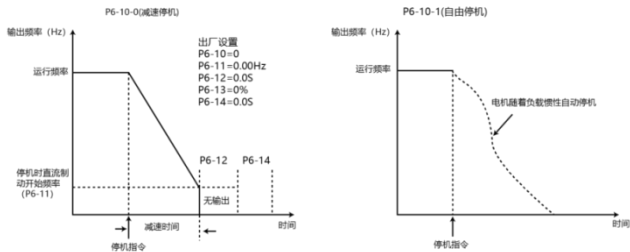
停机模式
