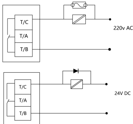
继电器输出端子抗干扰处理
