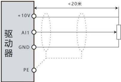
模拟量输入端子接线示意图
