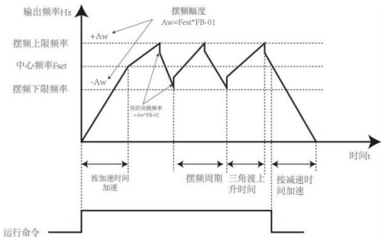
摆频工作示意图
