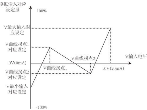
曲线4和曲线5示意图
