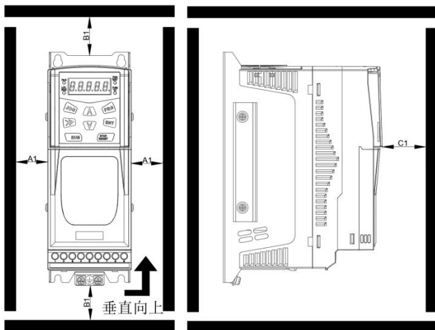
驱动器安装示意图
