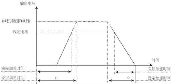
V/F分离示意图
