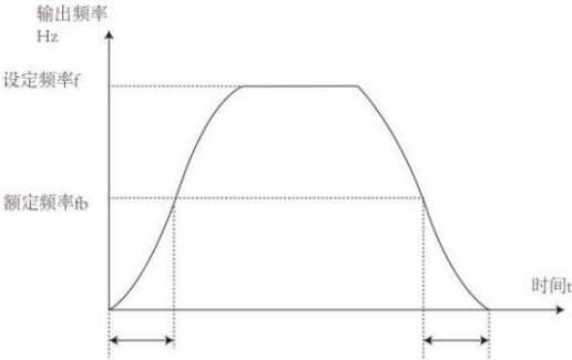
S曲线加减速B示意图
