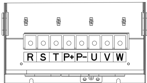
A6 主回路接线端子
