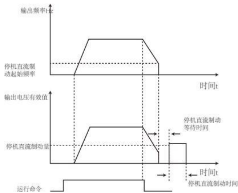
停机直流制动示意图
