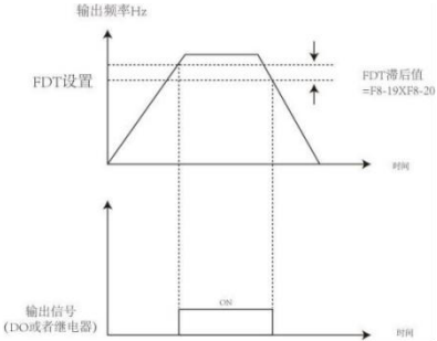
FDT电平示意图
