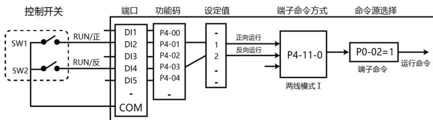
端子启停控制方式举例
