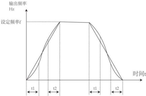
S曲线加减速A示意图
