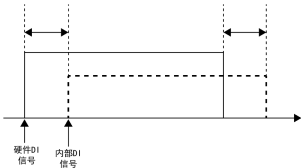
图6-19 DI 延迟设置
