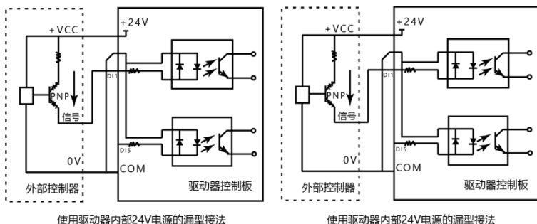
使用驱动器内部24V电源的漏型接法
