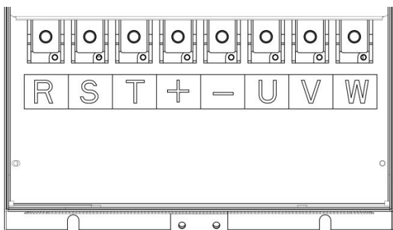
A8~A9主回路接线端子
