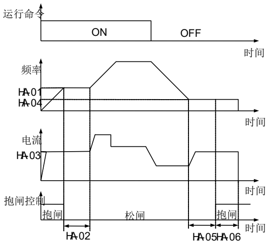
图.抱闸控制过程图
