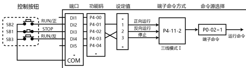
端子启停控制方式举例
