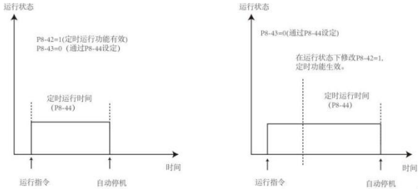
定时停机功能
