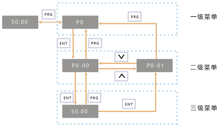
三级菜单操作流程图
