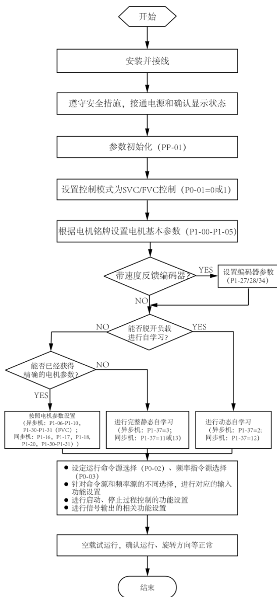
图7-3 FVC&amp;SVC调试流程
