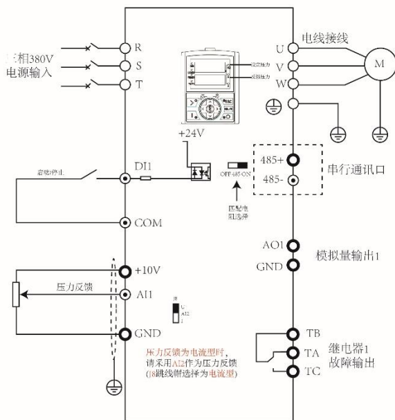
图1 压力反馈为电压型接线示意图
