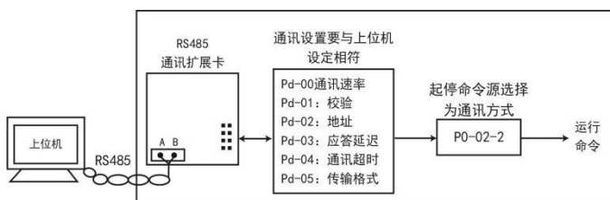
通讯启停控制方式举例
