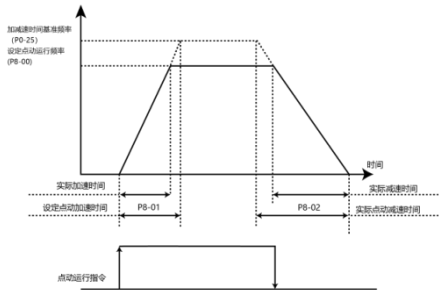
点动运行方式
