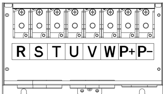
A7 主回路接线端子
