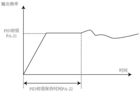
PID功能初值示意图
