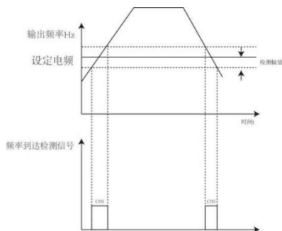
频率到达检测出幅值示意图
