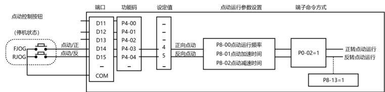
通讯S端口点动运行
