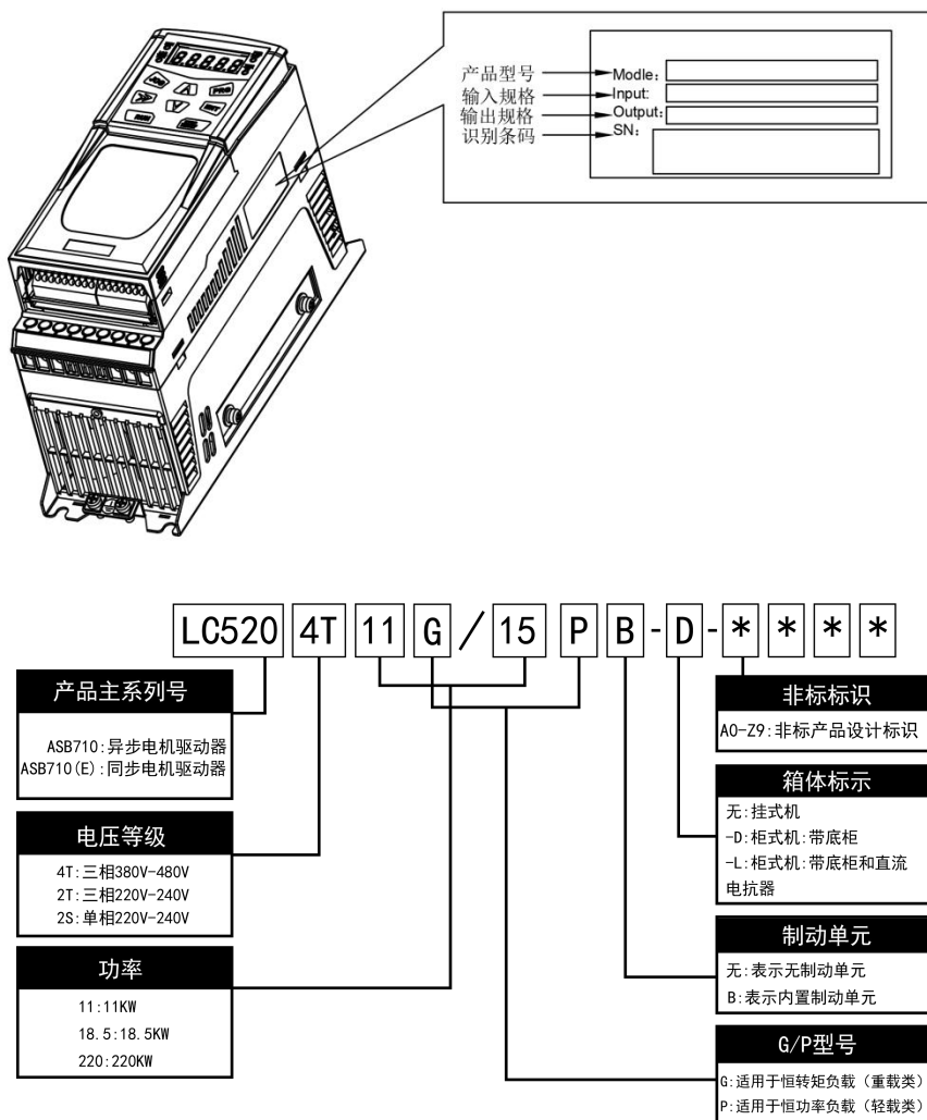
图2-2铭牌及产品命名
