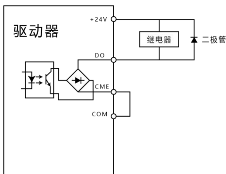
数字输出端子接线示意
